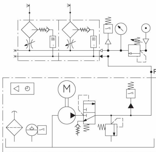
Installation avec une pompe électrique
